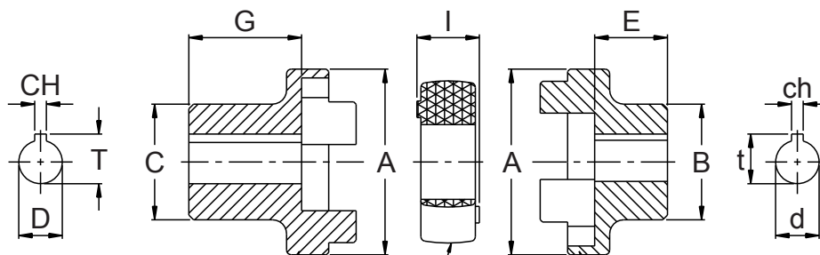
Accouplement usiné Type "ND"
