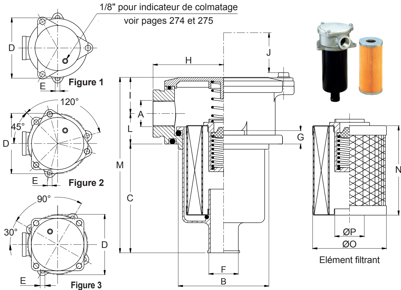
Filtre complet 25µ nom. Éléments filtrants 25µ nom.
