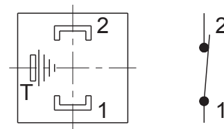
Branchement électrique
