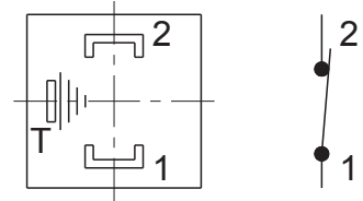
Branchement électrique
