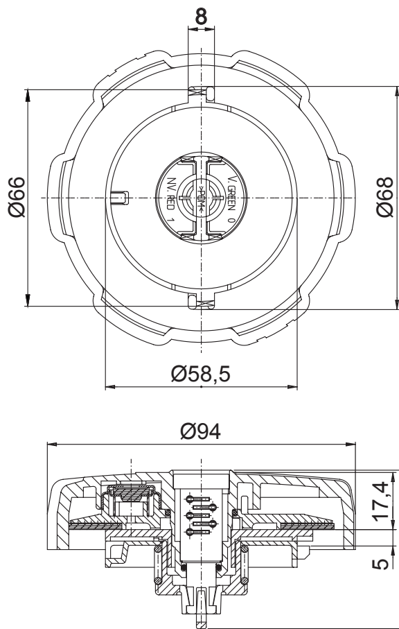
Bouchon 26521A
